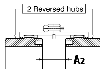
Fig. 03 - GO-ARR Coupling
